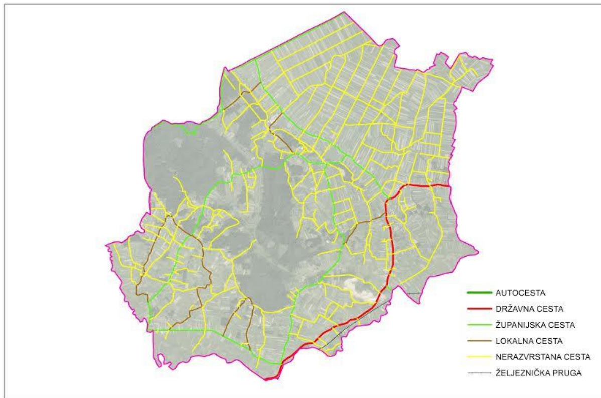
Slika 3: Mreža javnih i nerazvrstanih cesta na teritoriju Općine Maruševac
