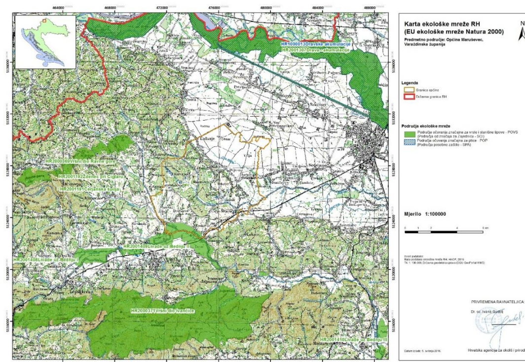
Slika 1: Područja Ekološke mreže NATURA 2000 na području Općine Maruševac
